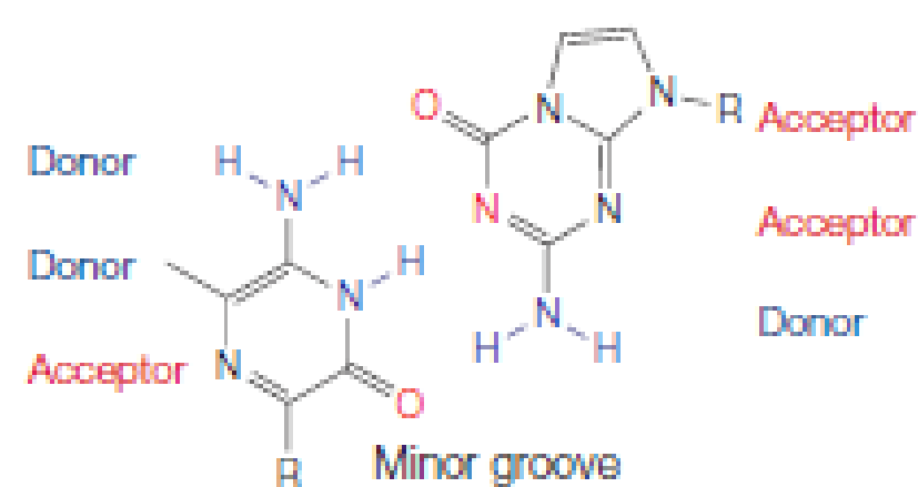
pyDDA
