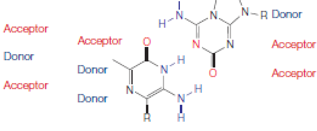
puADA
