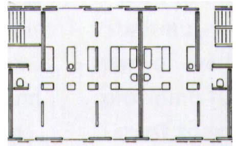
Abb.156 Graz-Sträßgang, Grundrisse
