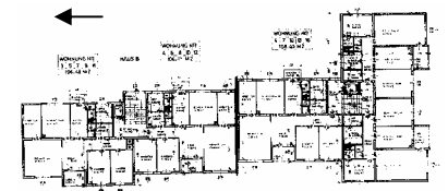
Abb.82 Geschossgrundriss Am Rehgrund
