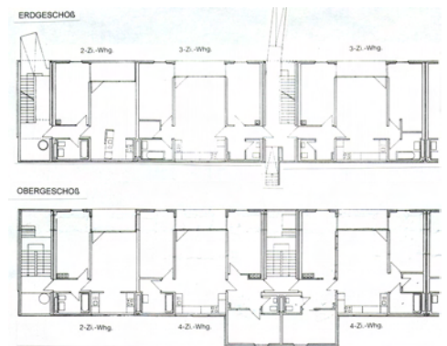
Abb.149 .Ziegelstrasse, Grundrisse
