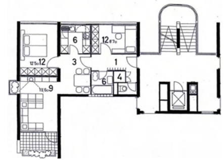
Abb.93 Hans Riehlgasse, Grundriss
