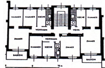
Abb.27. Dreispanner-Grundriss eines städtischen Wohnhauses nach 1923 mit Vorraum, Bad, WC, und 2-3 Zimmern !
