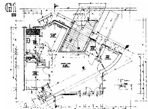
Abb.132 Neufeldweg, Grundriss
