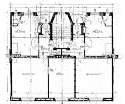
Abb.30. Grundriss Triestersiedlung I Vinzenz-Muchitsch-straße 1921
