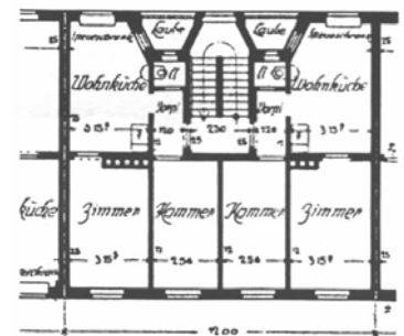
Abb. 30a München, Alte Haide, Grundriss, Theodor Fischer, 1919-23
