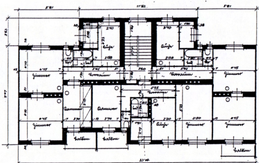
Abb. 1. Studie zu einem Typengrundriss.
