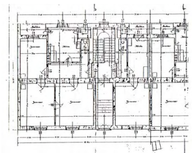
Abb.31.Grundriss Schönaugürtel 58-62
