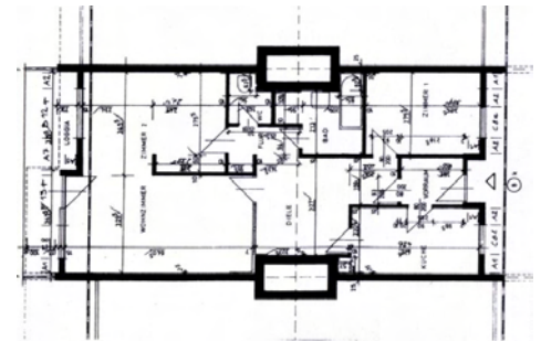
Abb.101 Terrassenhaussiedlung, Grundriss Typ i
