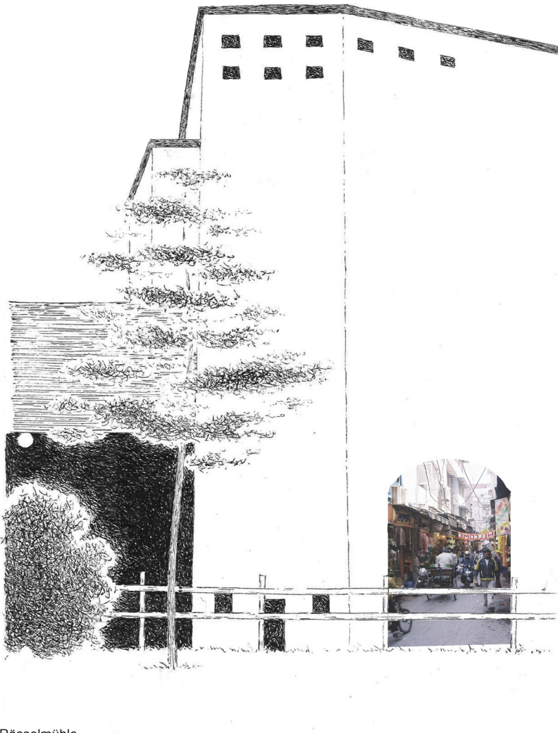
Rösselmühle
